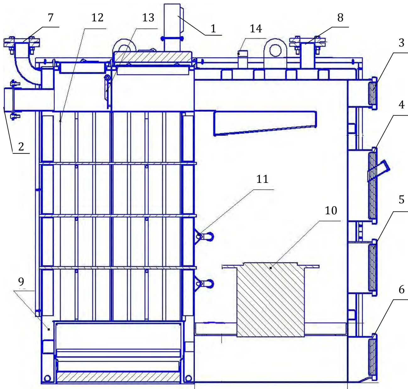
Конструкция котла рис. 4
