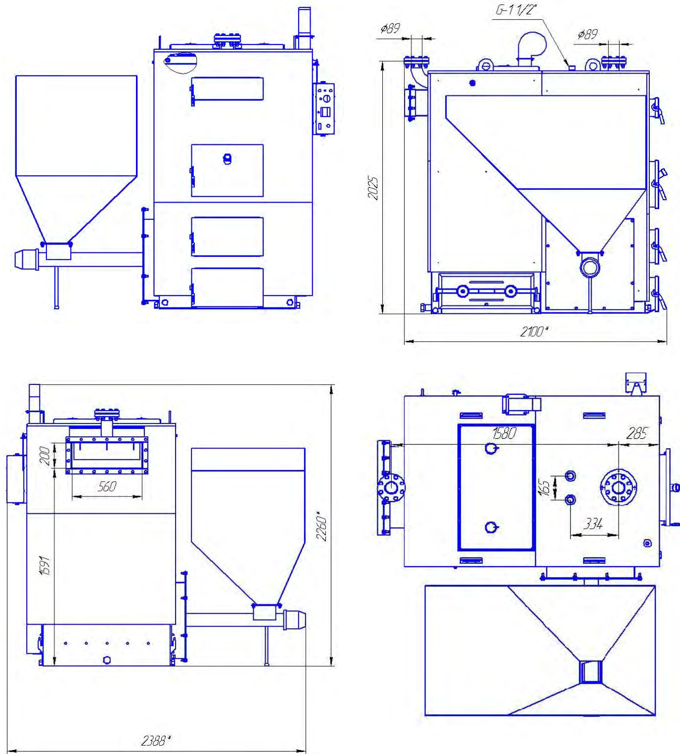
Установочный чертёж котла 200 WMSP рис. 2
