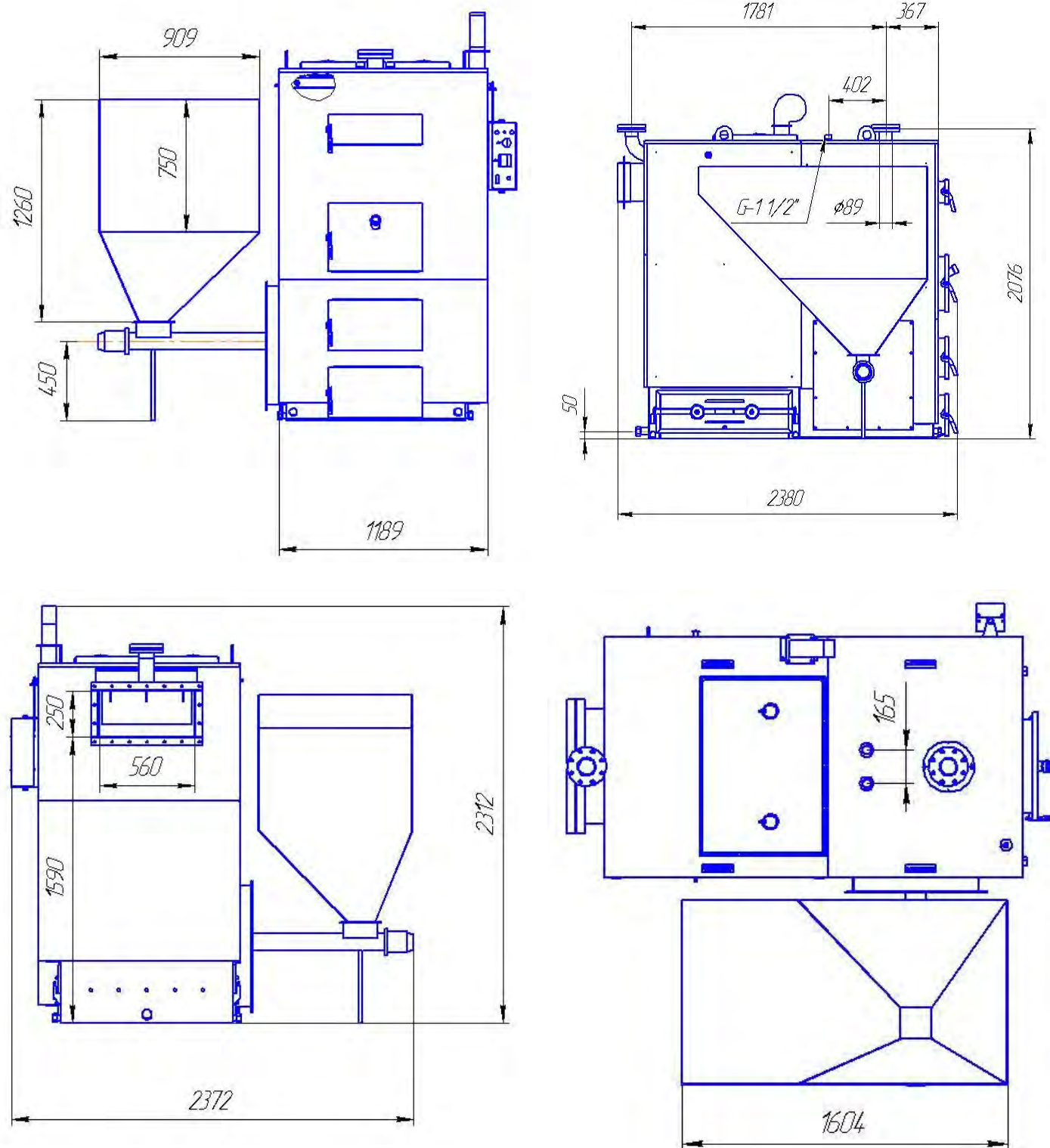
Установочный чертёж котла 250 WMSP рис. 3
